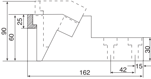
Ürün Nr. 2105 Blok Yandan Bağlama Product Nr. 2105 Block Side Press
