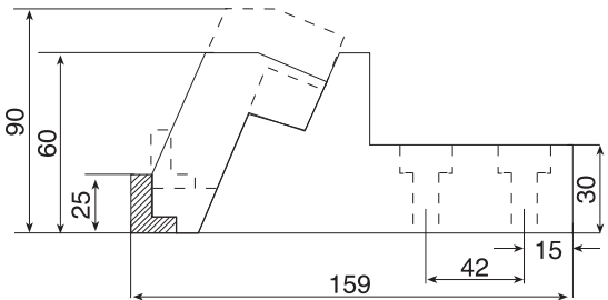
Ürün Nr. 2105 Blok Yandan Bağlama Product Nr. 2105 Block Side Press
