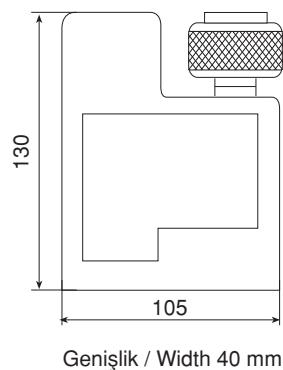
Ürün Nr. 1168 Kombine Bağlama Pabucu Alt Destek Product Nr. 1168 Combined Clamp Bottom Support
