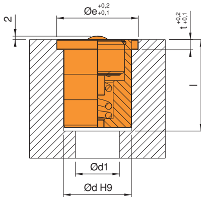
Ürün Nr. 1022 Yaylı Silindir Kalıp Kaldırma Model DBS Product Nr. 1022 Die Lifter Spring Cylinder Model DBS
