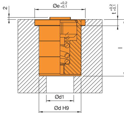
Ürün Nr. 1022 Yaylı Silindir Kalıp Kaldırma Model DLS Product Nr. 1022 Die Lifter Spring Cylinder Model DLS
