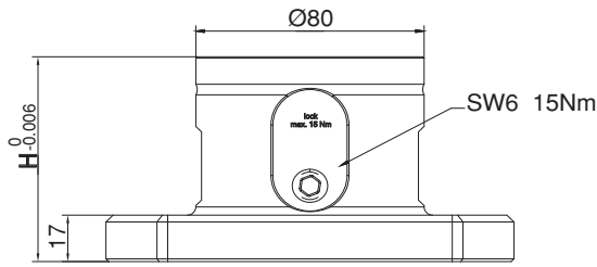
Ürün Nr. 0900 5-Eksen Blok Baęlama Product Nr. 0900 5-Axis Clamping Block
