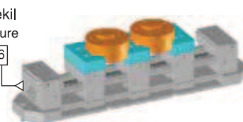
Yumuşak ayak ile bağlama şekli Figure clamping with soft legs
