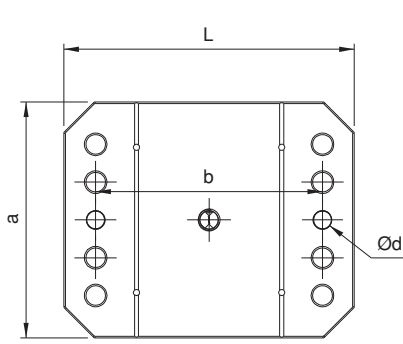
Ürün Nr. 2316 ER-EL Point Clamp
