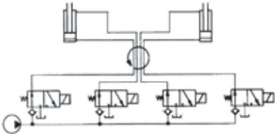
Hidrolik Devre Şeması Hydraulic Circuit Diagram
