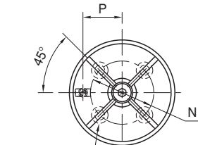
Gövde Sabitleme Civata Yuvası For Socket-Head Cap Screws
